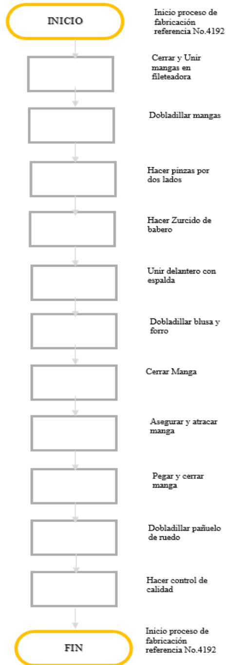
Figura 41. Flujograma de proceso de ensamble de una prenda de la referencia 4192
