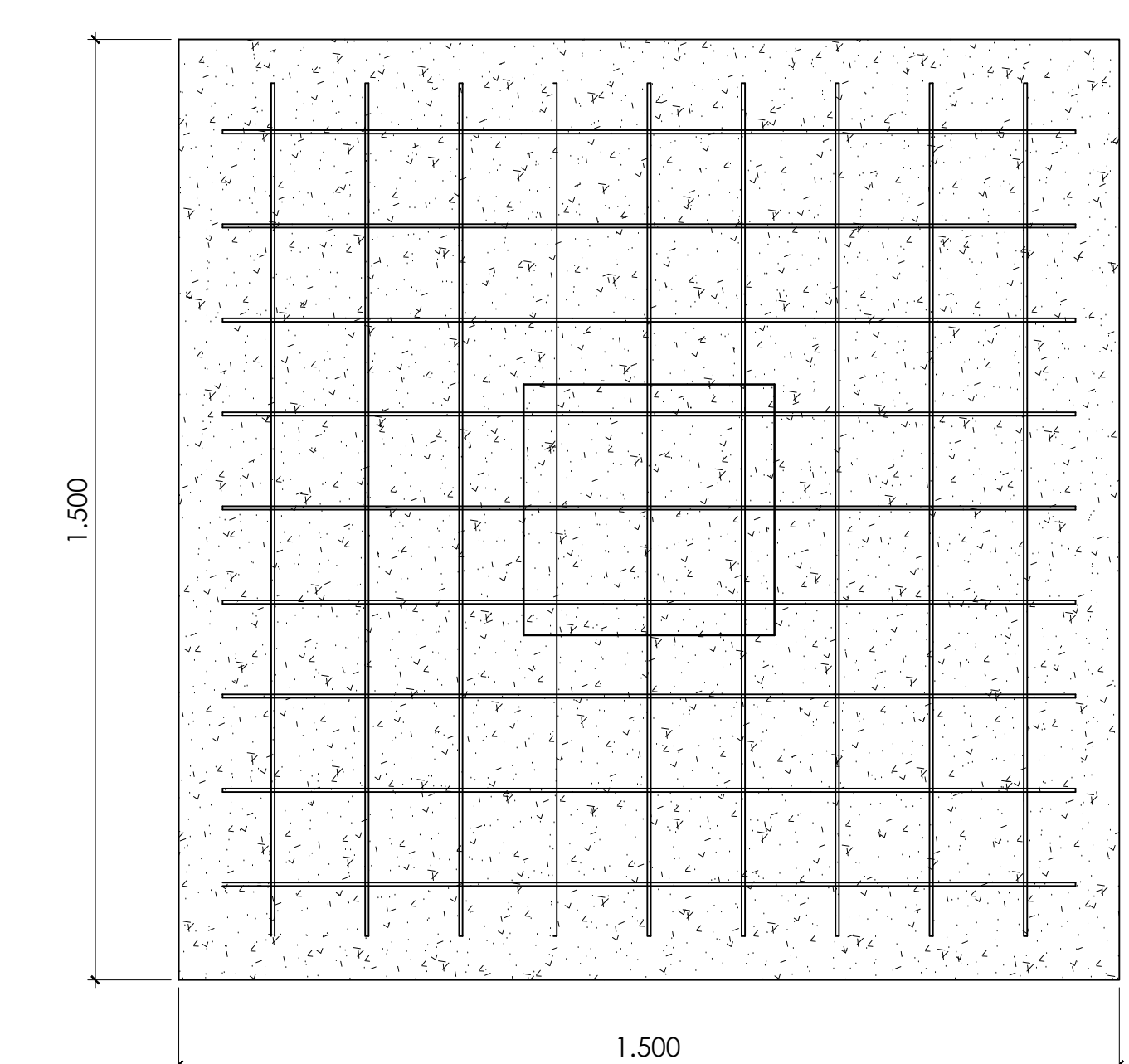
VISTA EN PLANTA DE ZAPATAS ESC. 1:10
