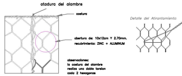
detalle de la costura malla del gabion escala 1:50
