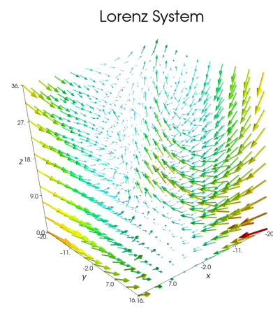
(d) Vector Field for equations 5.4
