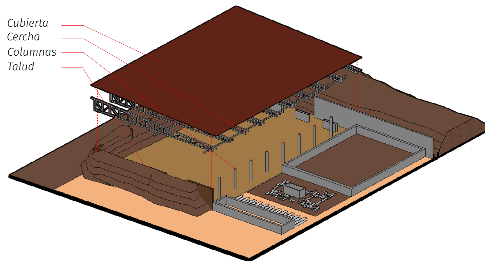
MODELO 3D - EXPLOTADO
