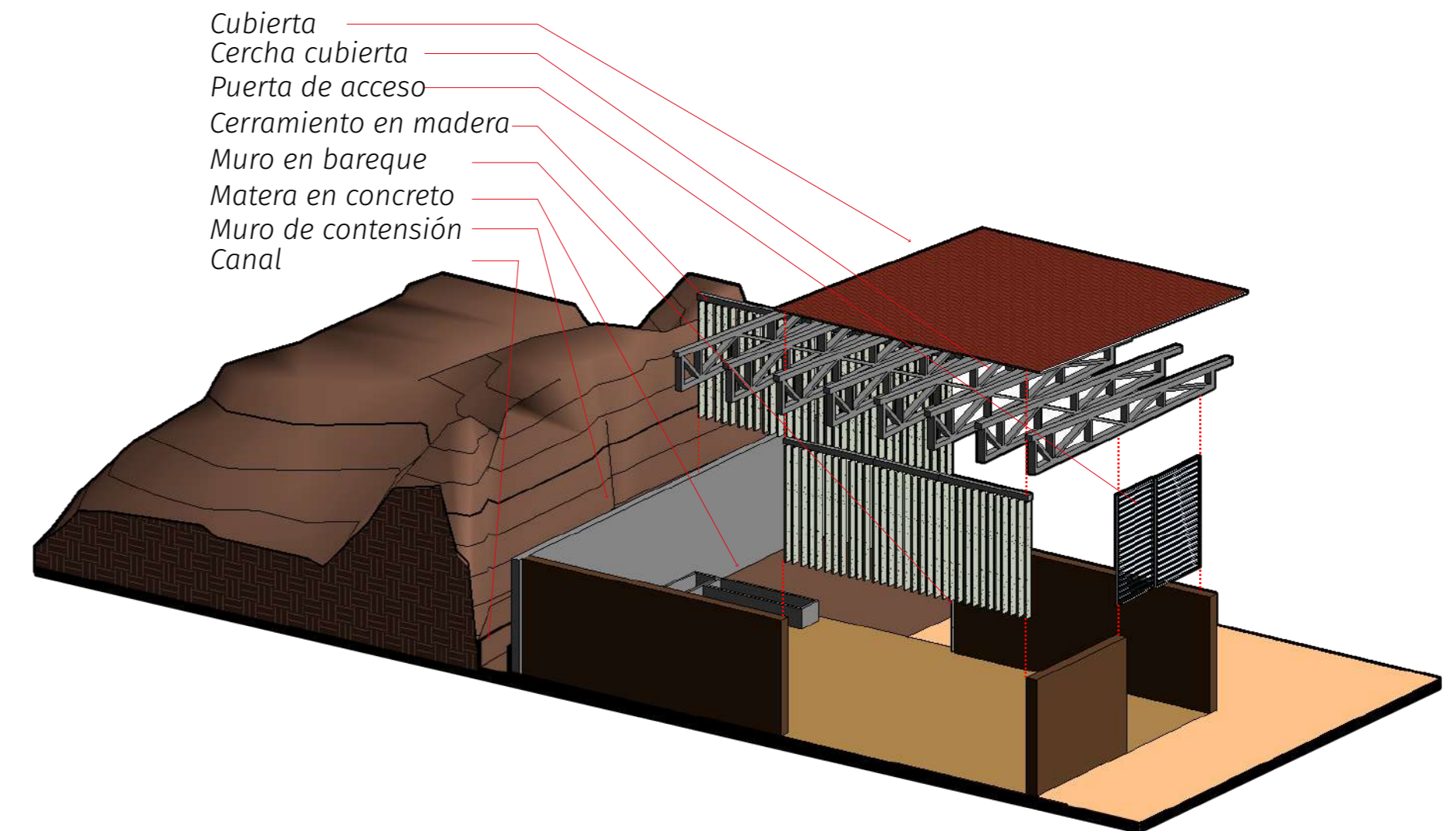
MODELO 3D - EXPLOTADO
