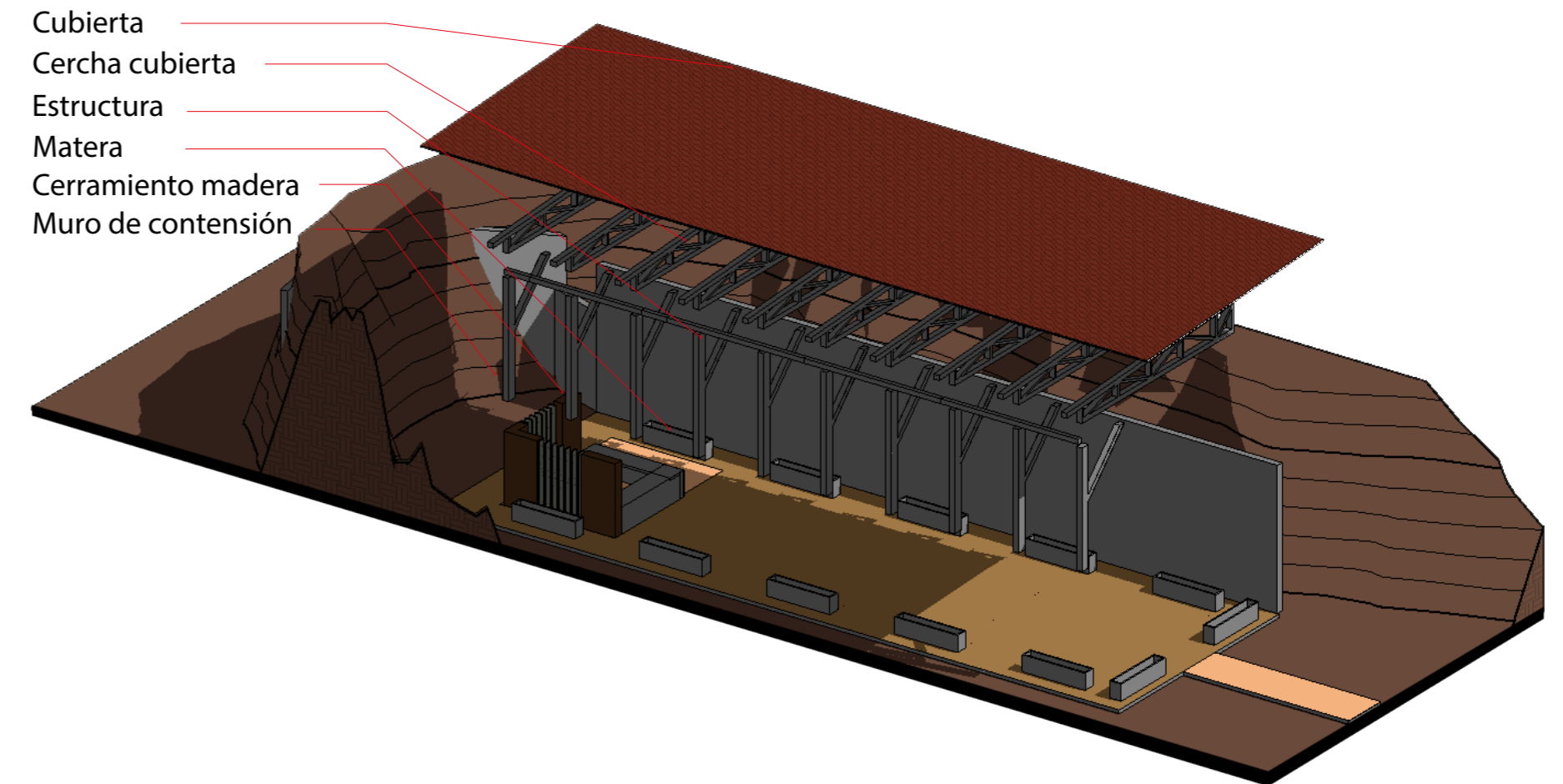
MODELO 3D - EXPLOTADO
