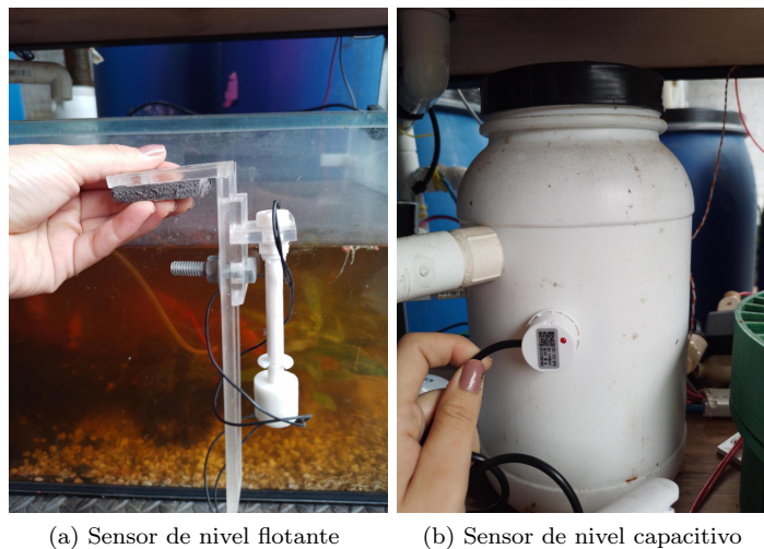
Figura 3.44: Sensores nivel
