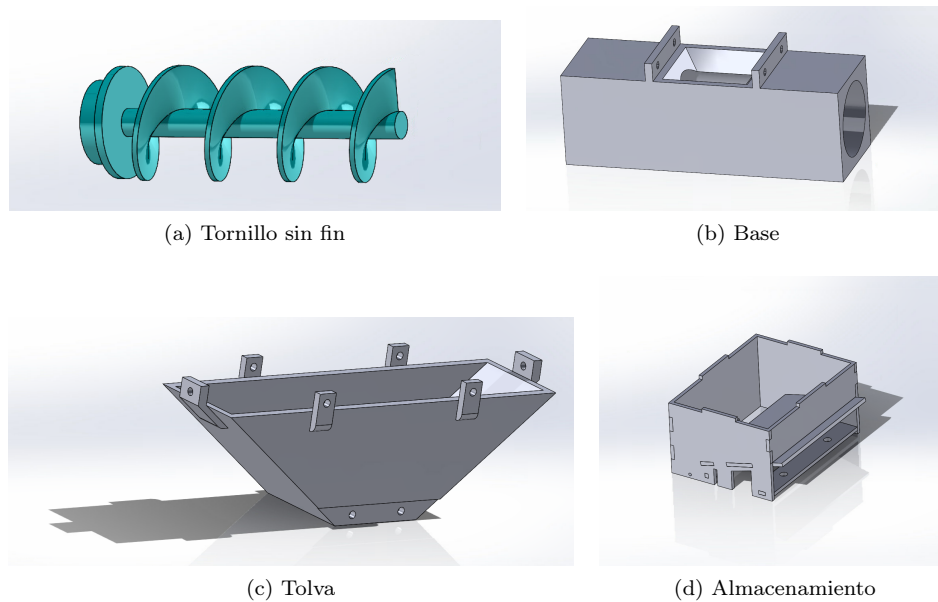
Figura 3.61: Partes de la primera versión del dosificador.
