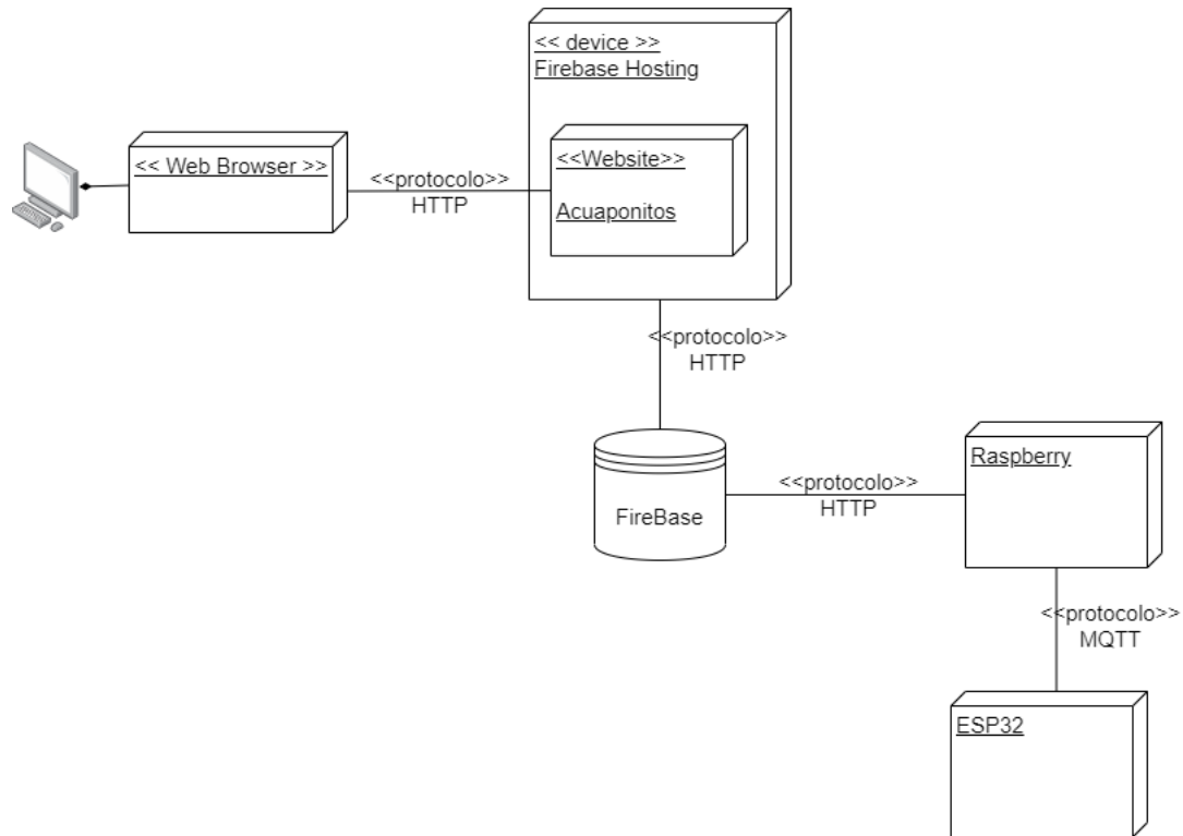
Figura 3.79: Arquitectura de ejecución
