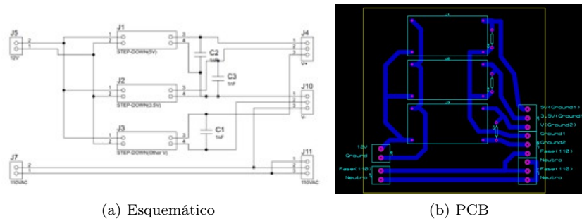
Figura 3.35: Esquemático y PCB - Módulo para convertidores
