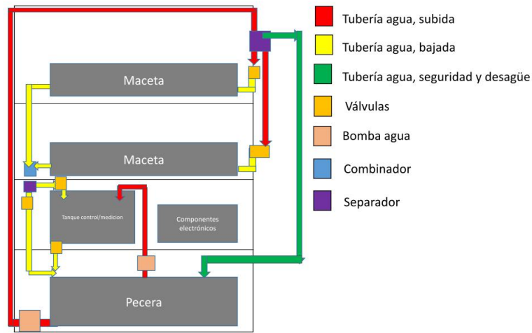
Figura 3.6: Vista frontal 2D de la estructura física con el flujo de agua
