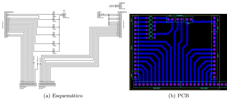
Figura 3.37: Esquemático y PCB - Módulo para relevos
