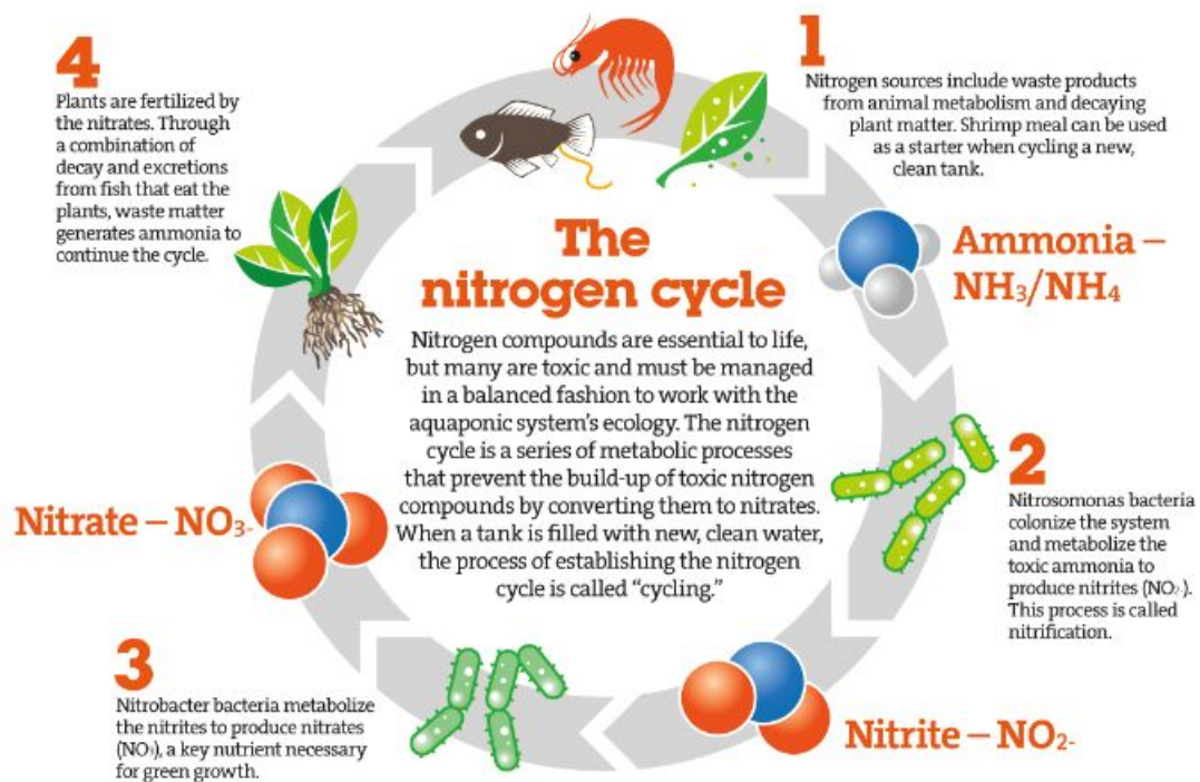
Figura 2.4: Proceso de nitrificación[38].
