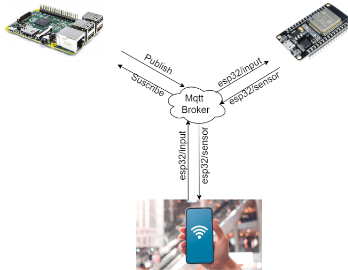
Figura 3.81: Arquitectura de red MQTT empleada en el proyecto de grado
