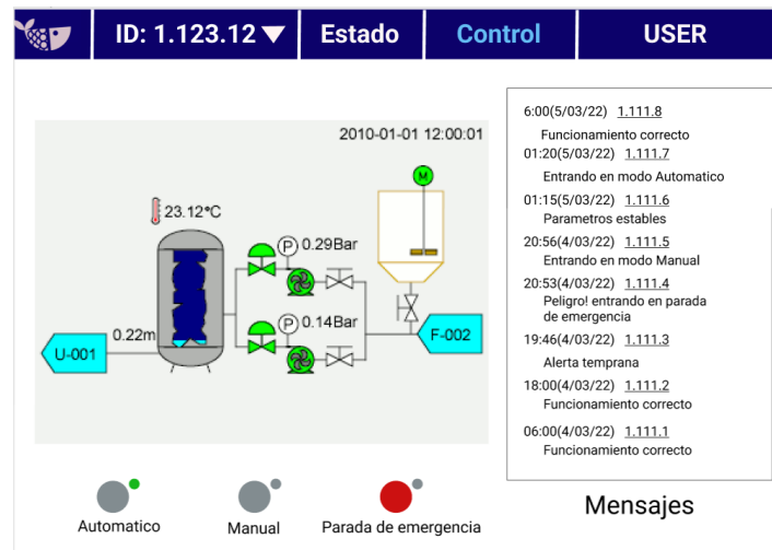
Figura 3.72: Diseño de vista control
