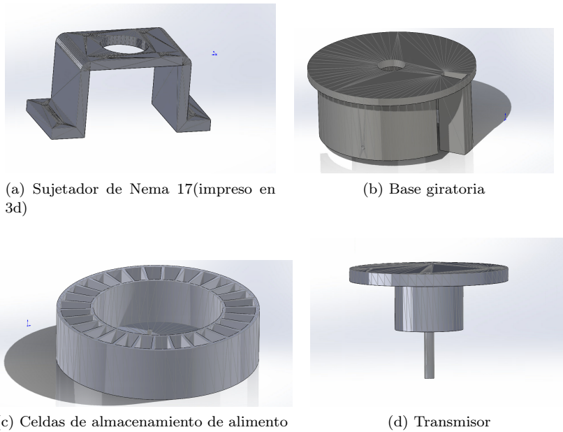
Figura 3.63: Partes de la segunda versión del dosificador.
