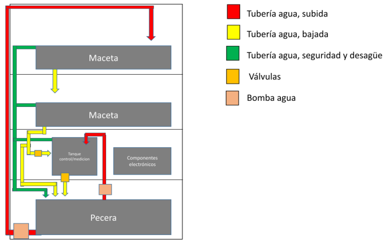
Figura 3.14: Vista frontal 2D de la estructura física con el rediseño del flujo de agua
