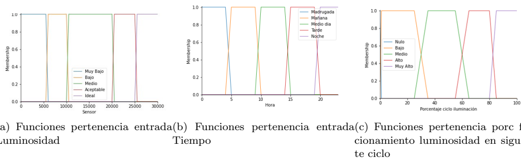
Figura 3.85: Funciones de pertenencia
