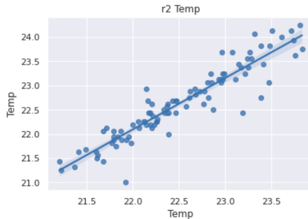
Figura 3.89: Resultados de evaluación de predicción de temperatura empleando control moderno
