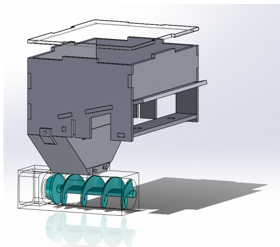
Figura 3.60: Diseño de tolva dosificadora con tornillo sin fin accionada por nema 17
