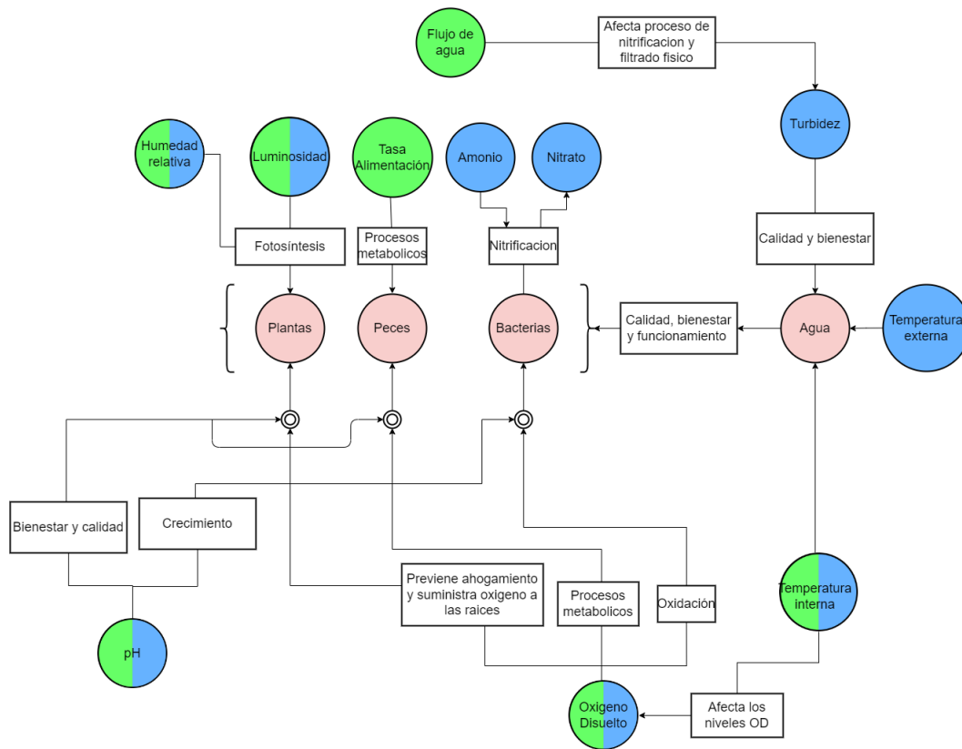
Figura 2.6: Árbol de interacciones entre variables del sistema acuapónico
