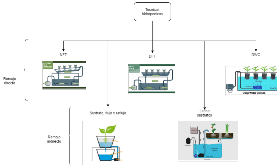
Figura 2.3: Técnicas hidróponicas.[8, 31, 32]
