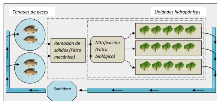
Figura 2.5: Partes de un sistema acuapónico [39].
