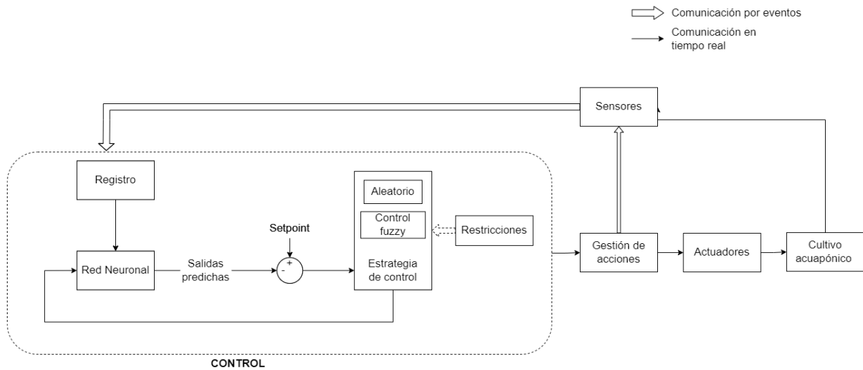
Figura 3.82: Arquitectura de control
