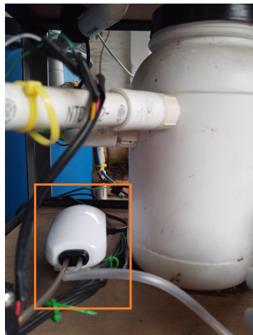
Figura 3.64: Bomba de aire
