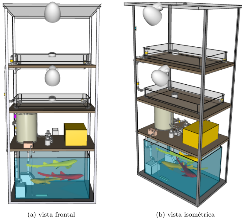
Figura 3.5: Diseño de la estructura en software CAD
