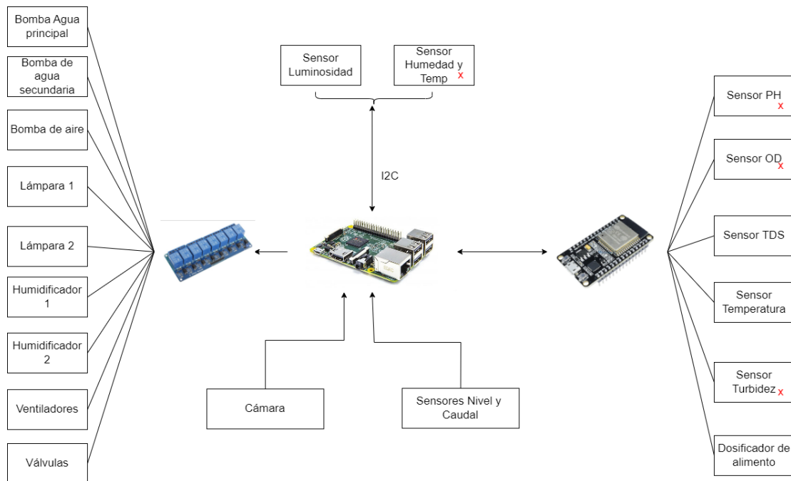
Figura 3.19: Diagrama de conexiones principales
