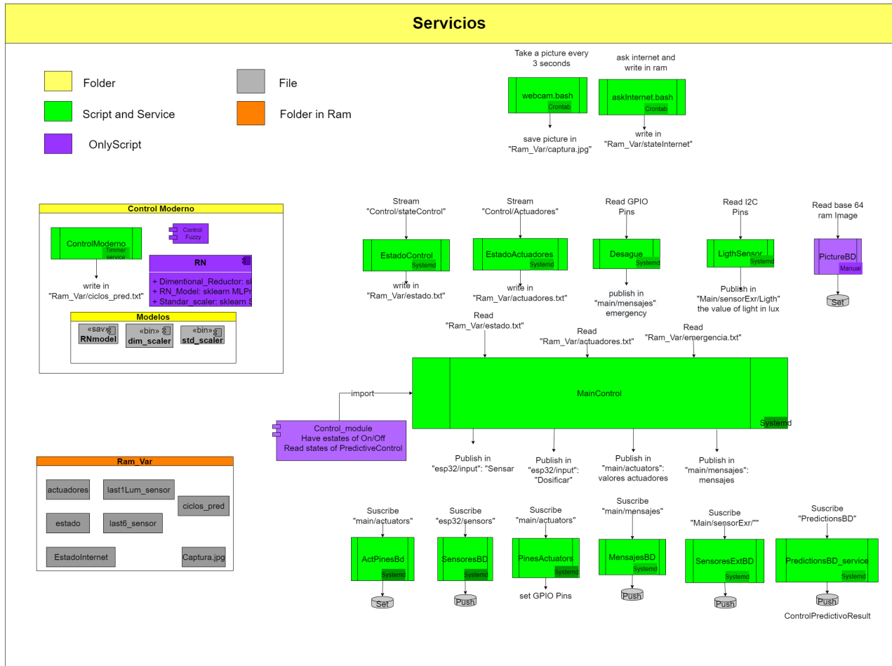
Figura 3.93: Diagrama de servicios construidos
