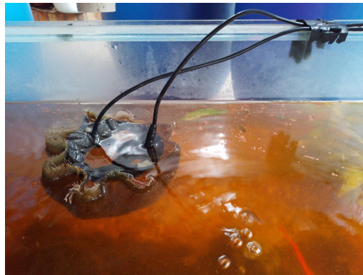
Figura 3.43: Instalación final de los sensores con malla de protección.
