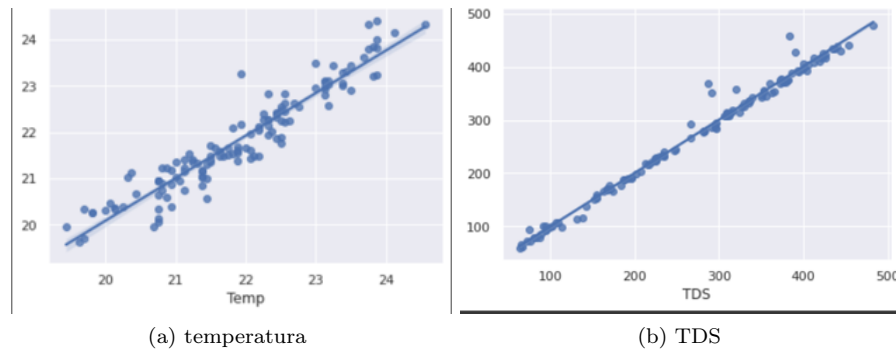
Figura 3.87: Resultados de evaluación mediante coeficiente de determinación
