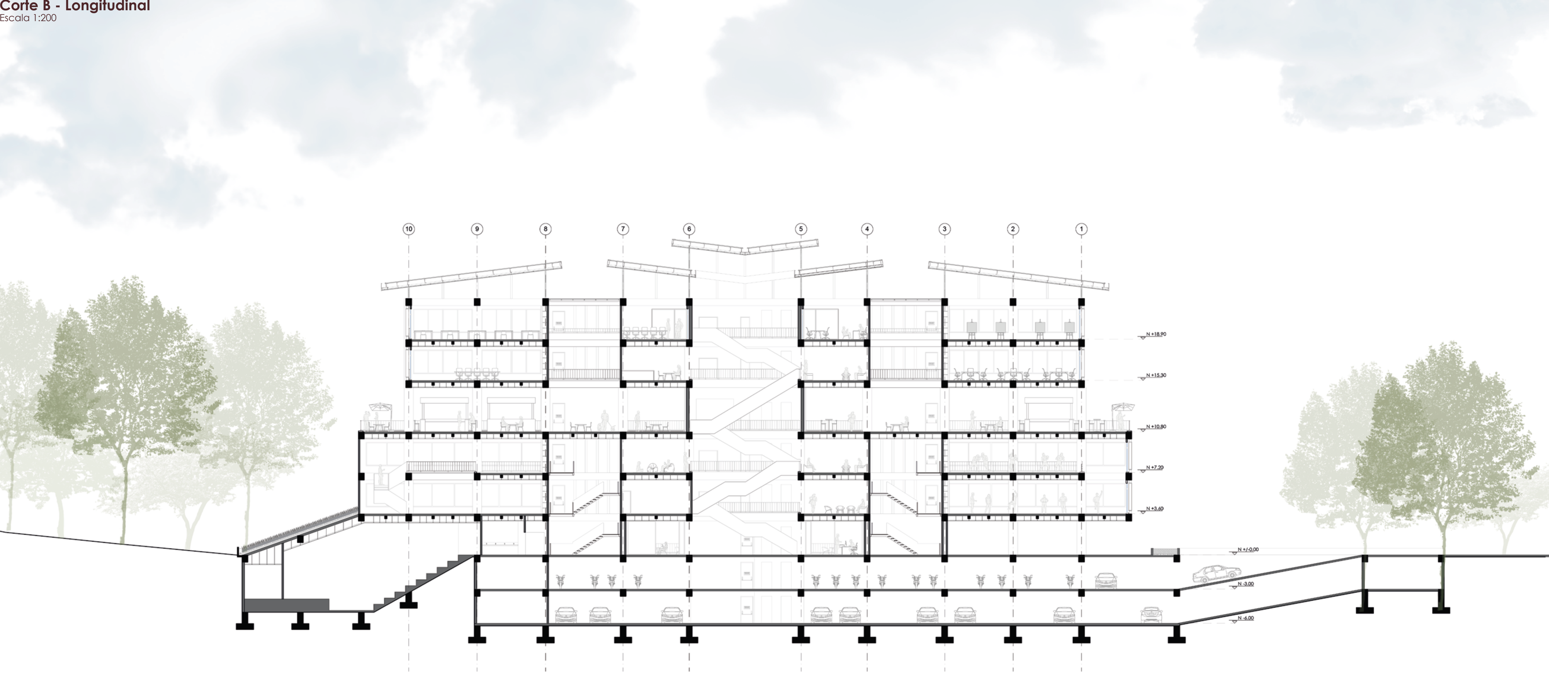
Corte B - Longitudinal
