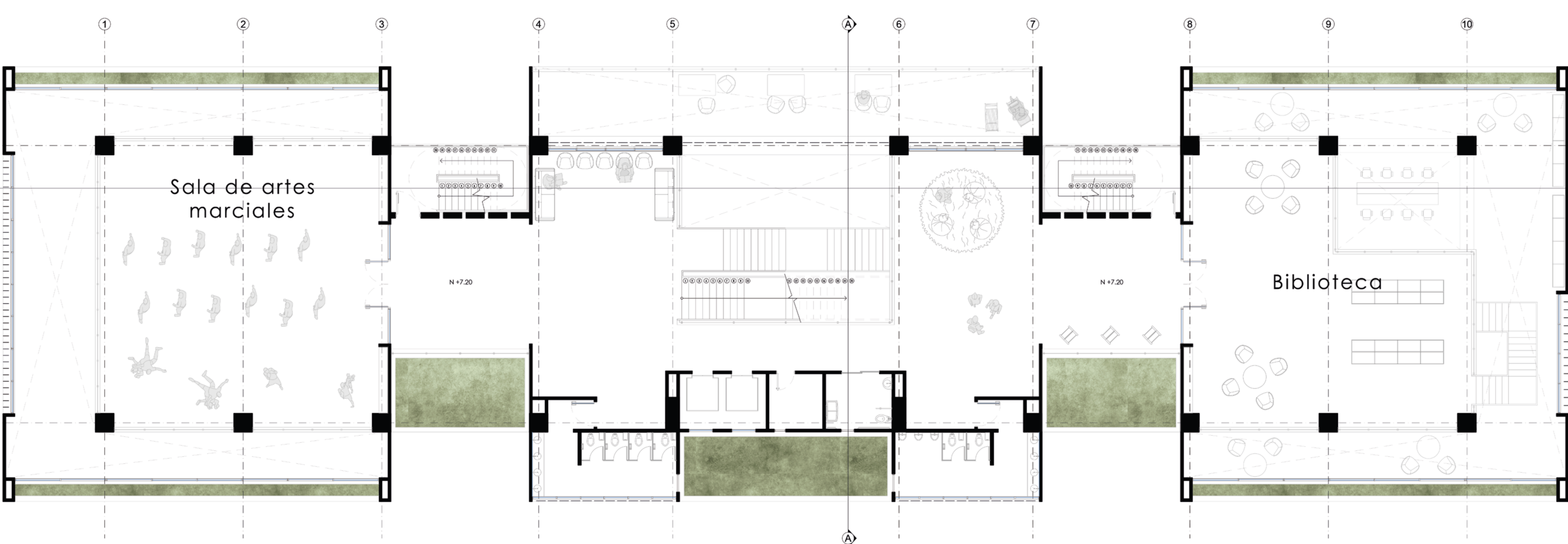
Planta Piso 5 N +15.30
