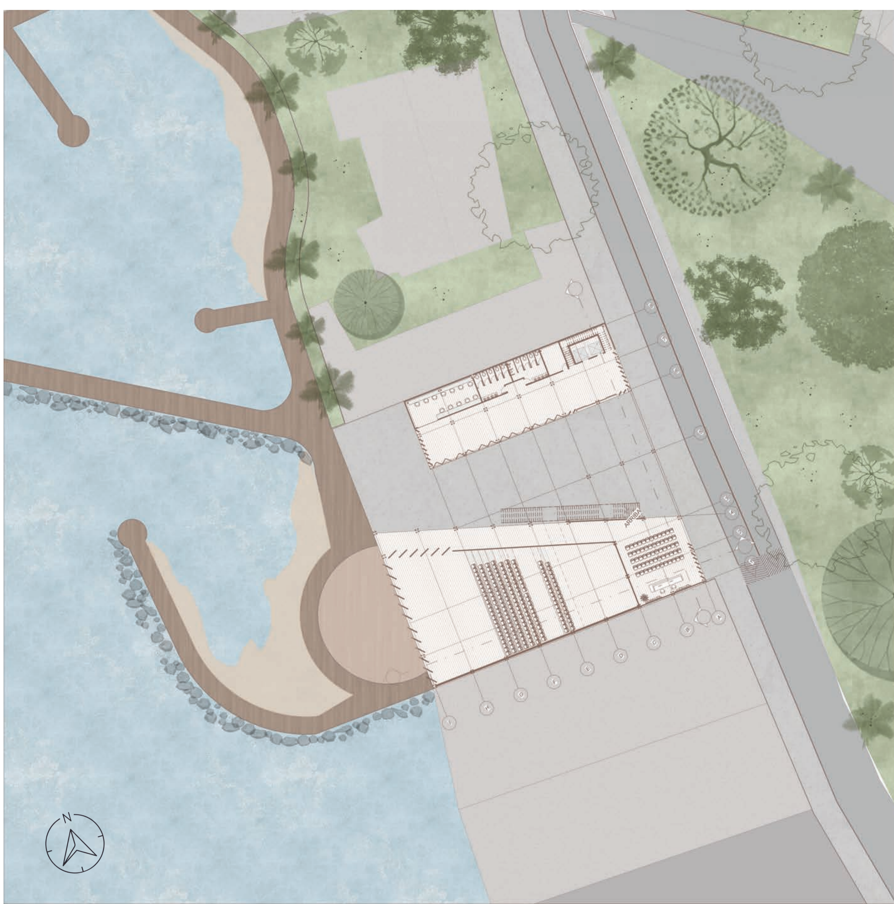
PLANTA PÚBLICA ESC. 1:250
