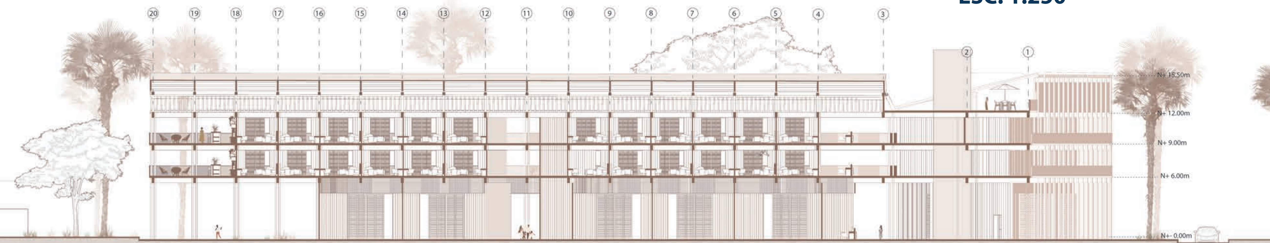
CORTE TRANSVERSAL ESC. 1:250
