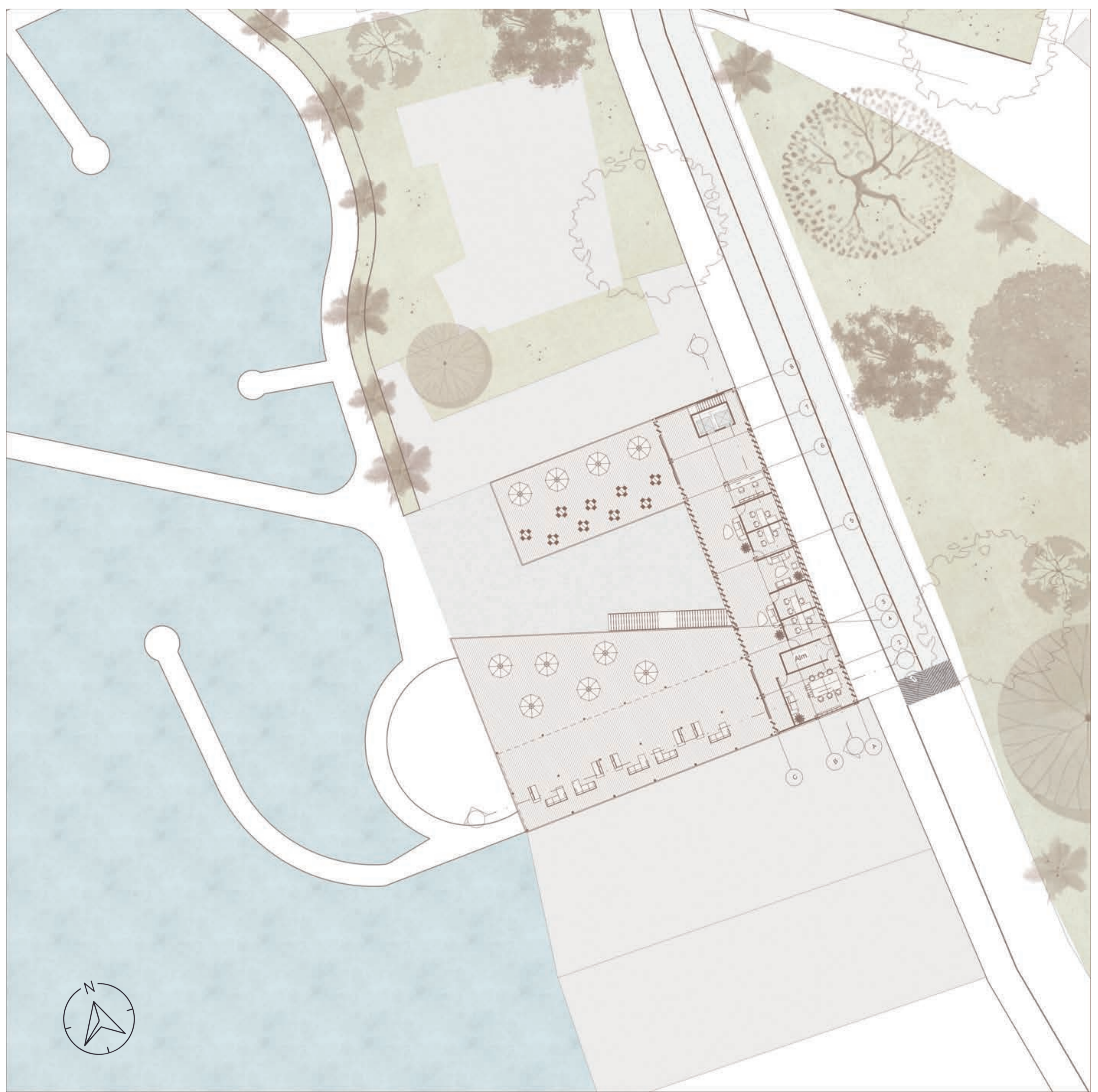
PLANTA TIPO PISO 3 ESC. 1:250
