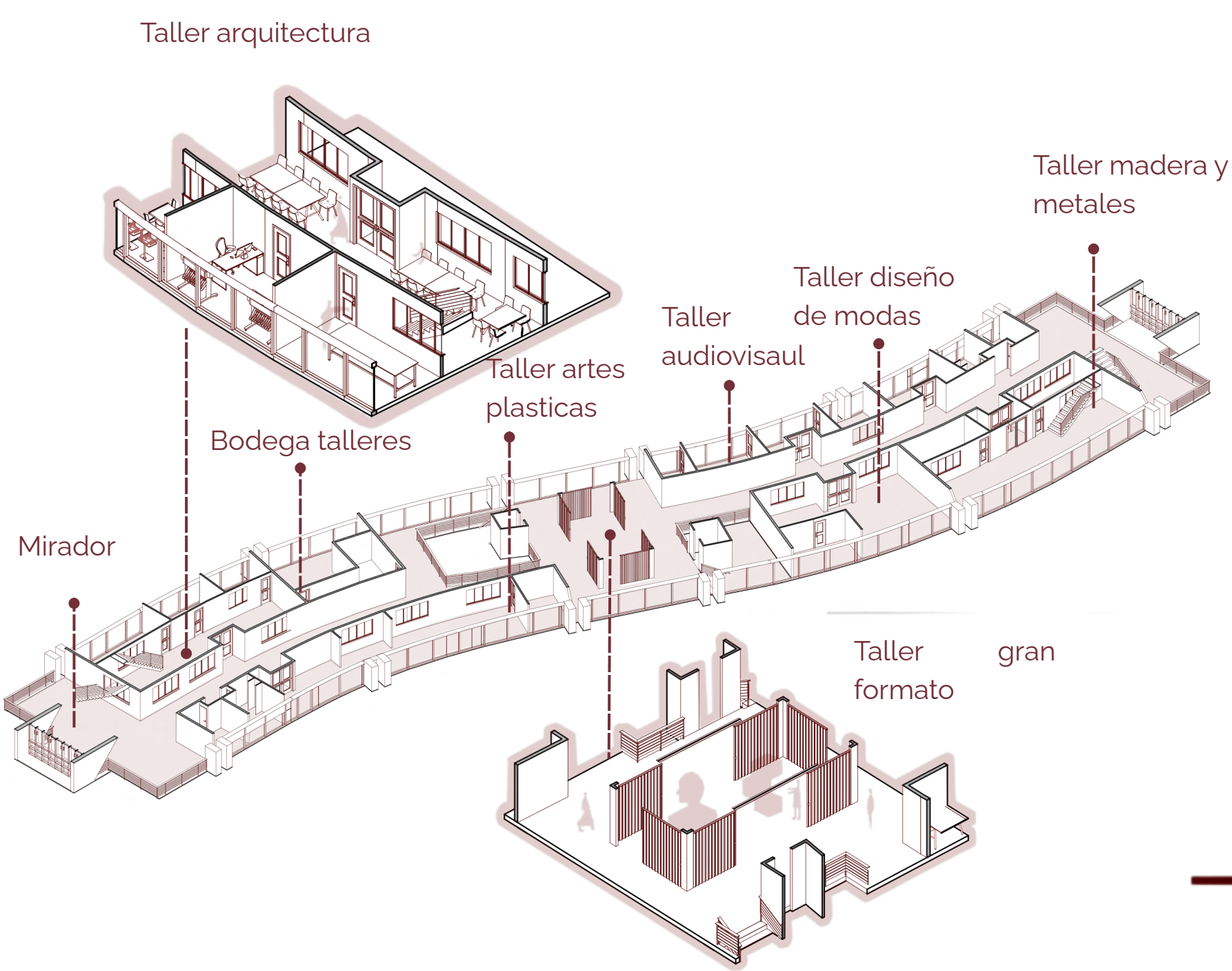
03 SEGUNDA PLANTA ESC 1: 200
