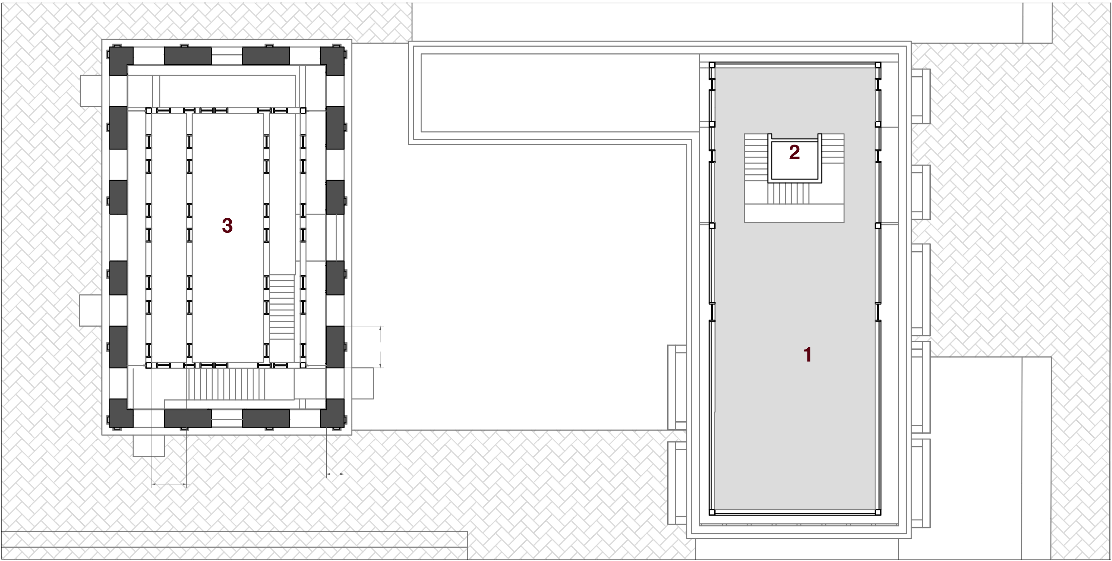
PLANTA 4 1. Administración 2. Punto fijo 3. Torre simbólica el molino
