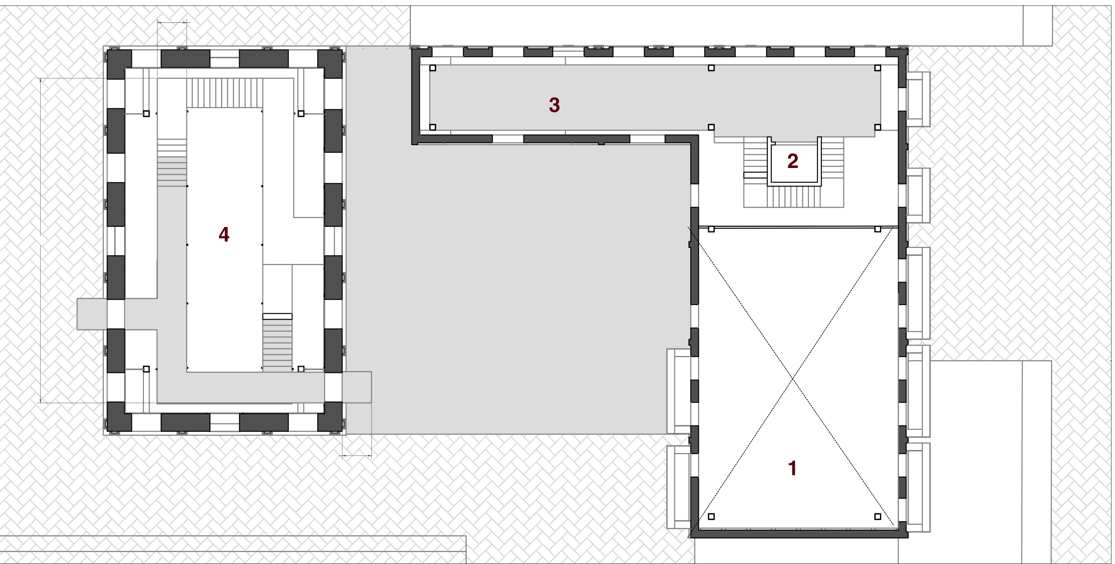
PLANTA 2 1. Zona para exposiciones 2. Punto fijo 3. Zona comercial 4. Torre simbólica el molino
