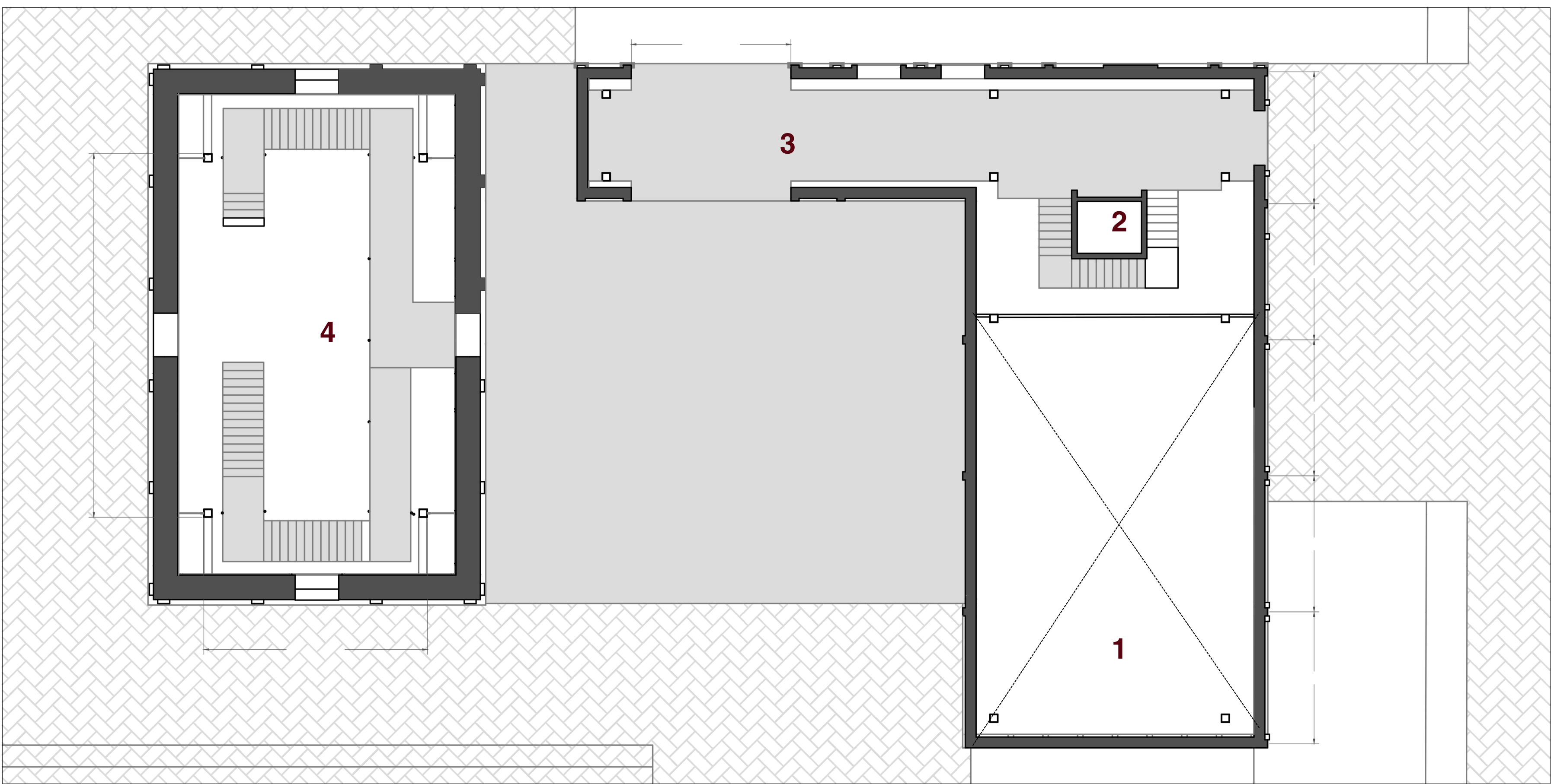
PLANTA 1 1. Zona para exposiciones 2. Punto fijo 3. Zona comercial 4. Torre simbólica el molino
