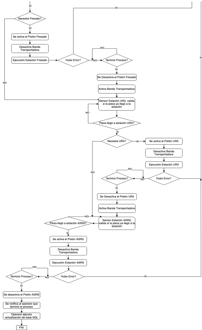
Figura 6.10: Lógica Funcional Celda de manufactura CAP Parte 2
