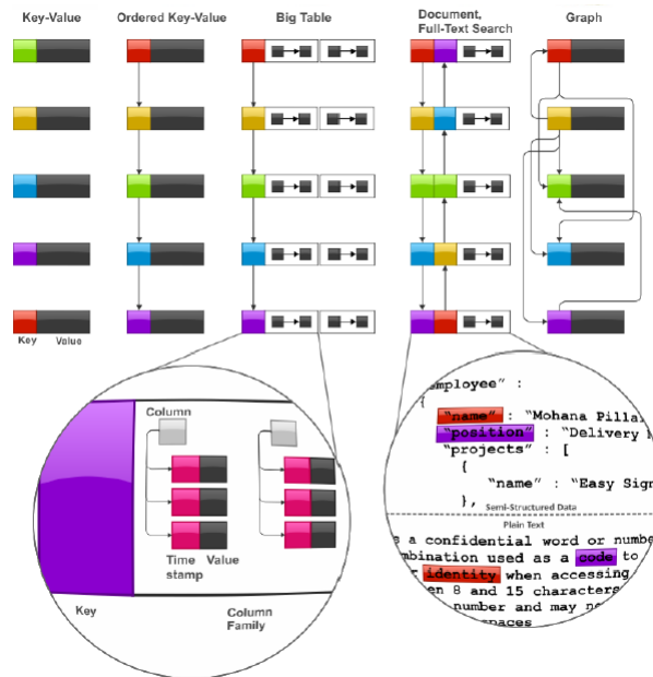
Figura 5.3: Bases de datos NoSQL[3].
