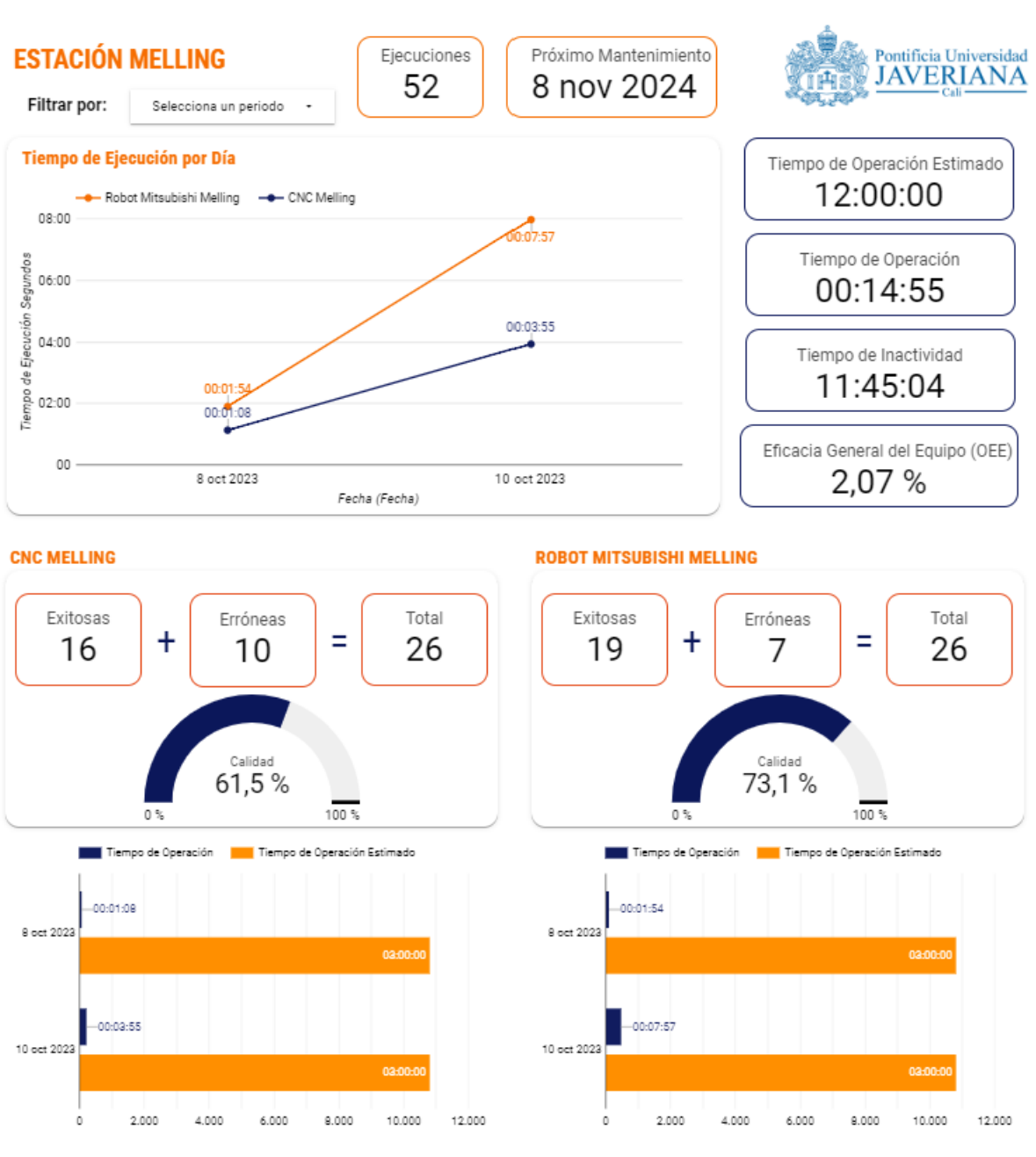
Figura 8.9: Reporte de Estación Fresado
