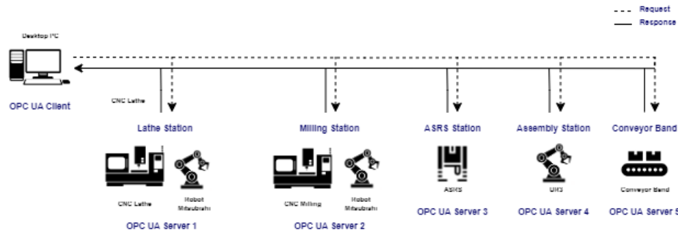
Figura 6.8: Diagrama de comunicación OPC UA Celda de Manufactura del CAP
