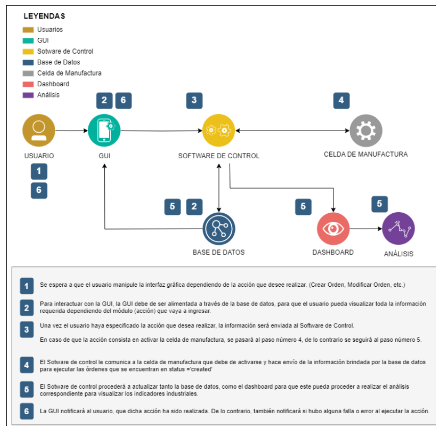
Figura 8.1: Boceto Comunicación Componentes del Sistema de Información
