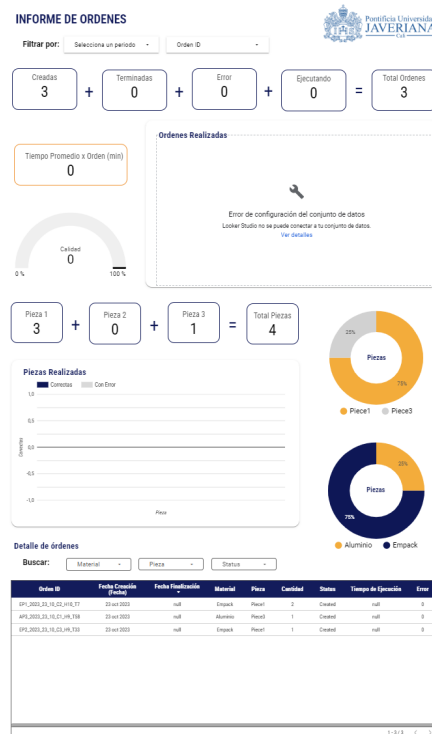
Figura 8.28: Actualización Dashboard
