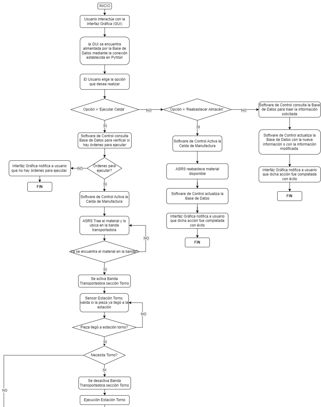
Figura 8.16: Lógica funcional Software de Control Parte 1
