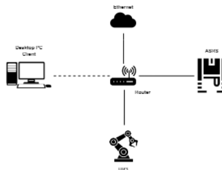
Figura 6.7: Diagrama de Comunicación Ethernet Celda de Manufactura del CAP
