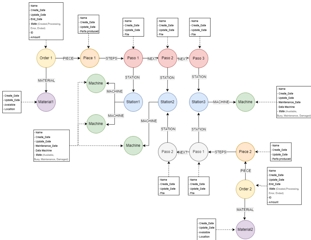
Figura 7.3: Boceto No.3 Base de Datos
