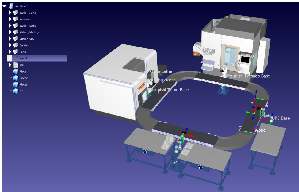
Figura 8.14: Celda de Manufactura en RoboDK
