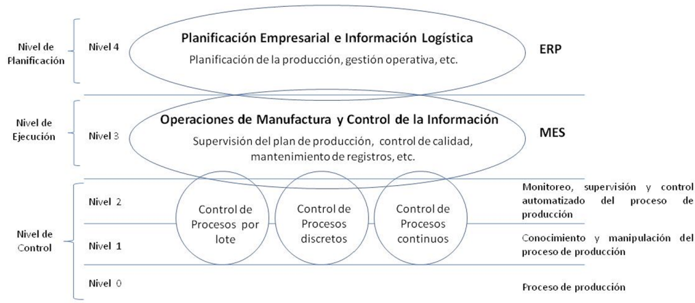
Figura 5.1: Jerarquía Funcional sistema MES.[1]
