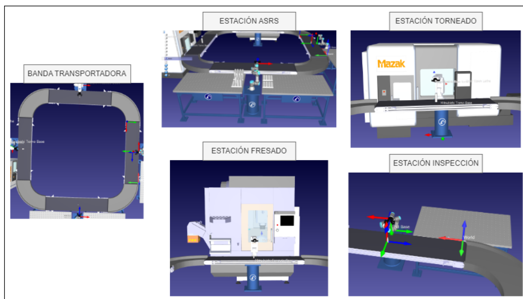
Figura 8.15: Estaciones en RoboDK
