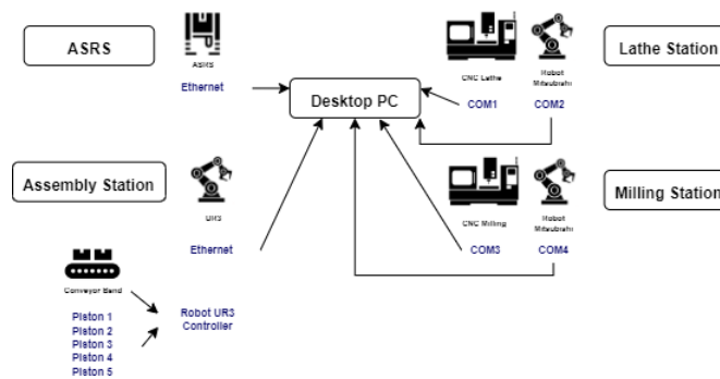
Figura 6.6: Diagrama Global de la Celda de Manufactura del CAP
