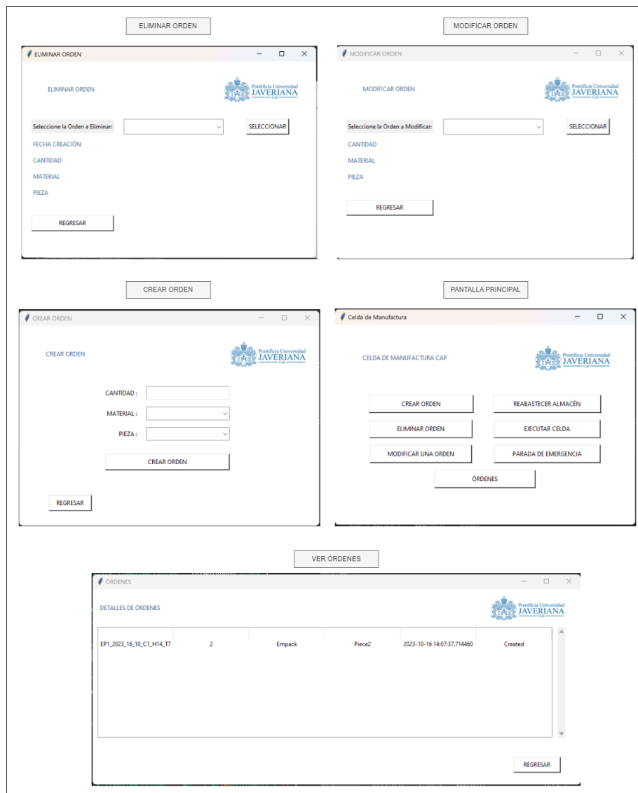
Figura 8.13: Interfaz Gráfica GUI desarrollada en Tkinter Python
