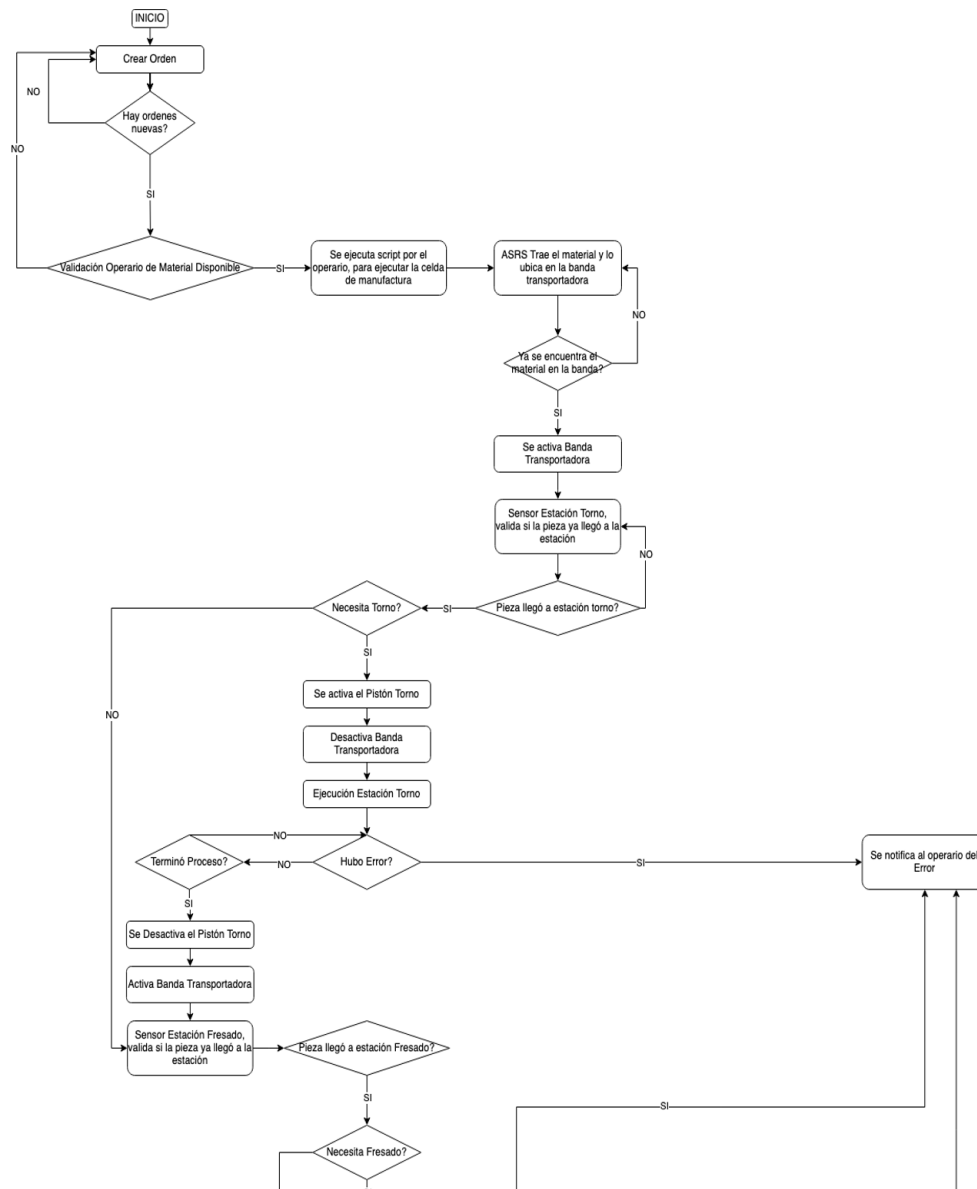
Figura 6.9: Lógica Funcional Celda de manufactura CAP Parte 1
