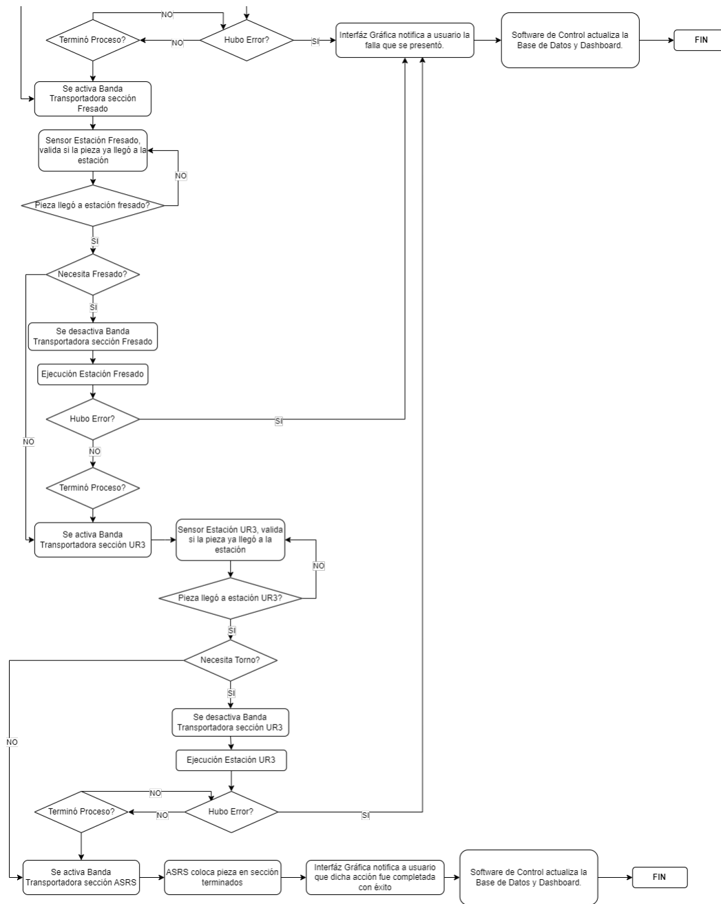
Figura 8.17: Lógica funcional Software de Control Parte 2
